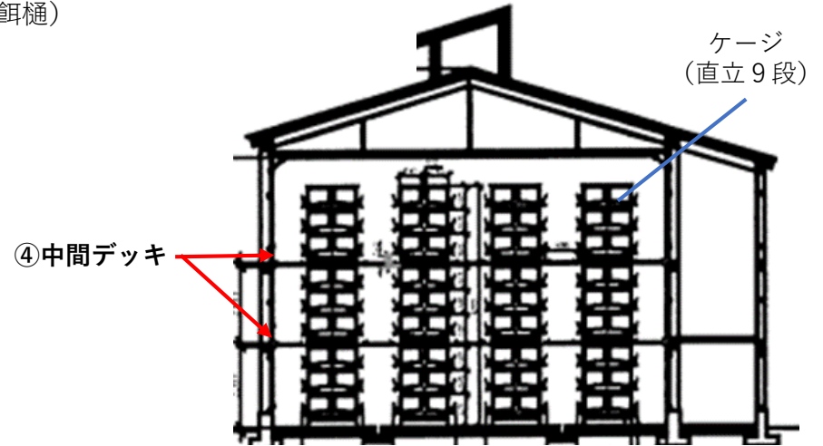
○鶏舎断面図
