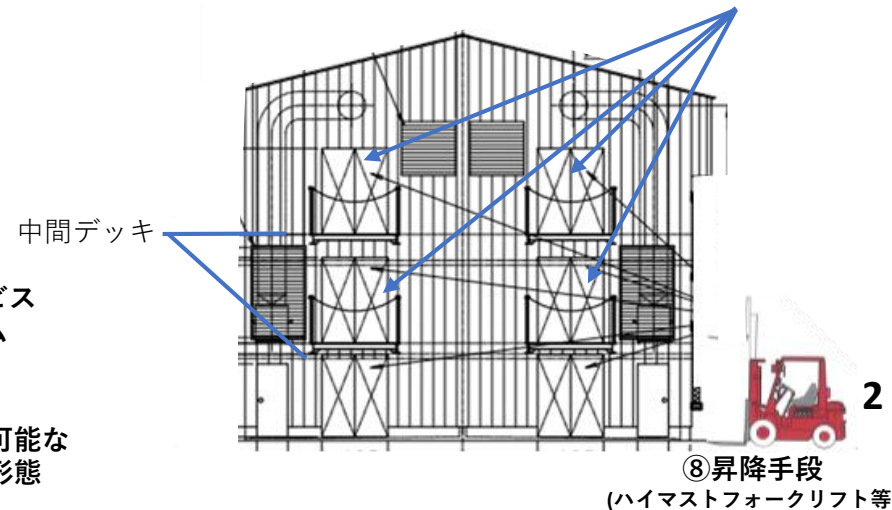
○鶏舎外観図
