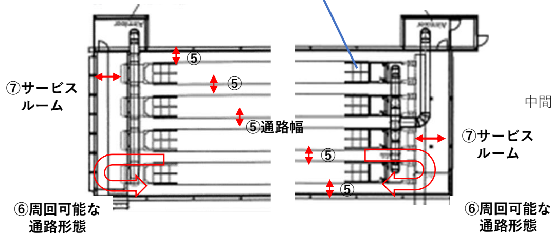
○鶏舎平面図
